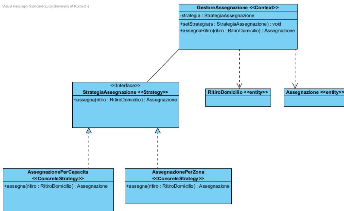
Figura 48: Struttura UML del Design Pattern Strategy per l'allocazione delle risorse
