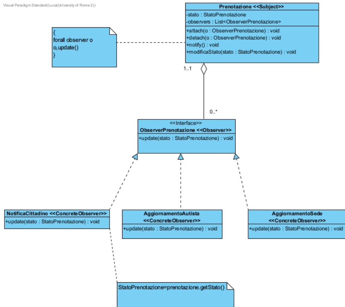
Figura 47: Struttura UML del Design Pattern Observer applicato a MyAma
